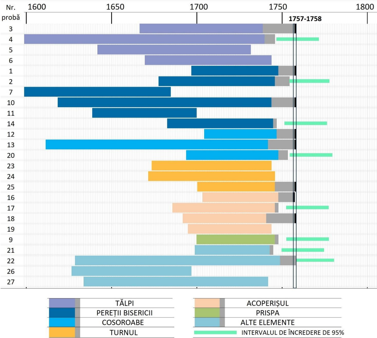
Graficul nr. 3. Biserica de lemn din Bulgari. Intervalul temporal acoperit de fiecare dintre probele date (cu gri sunt indicate inelele de alburn).
