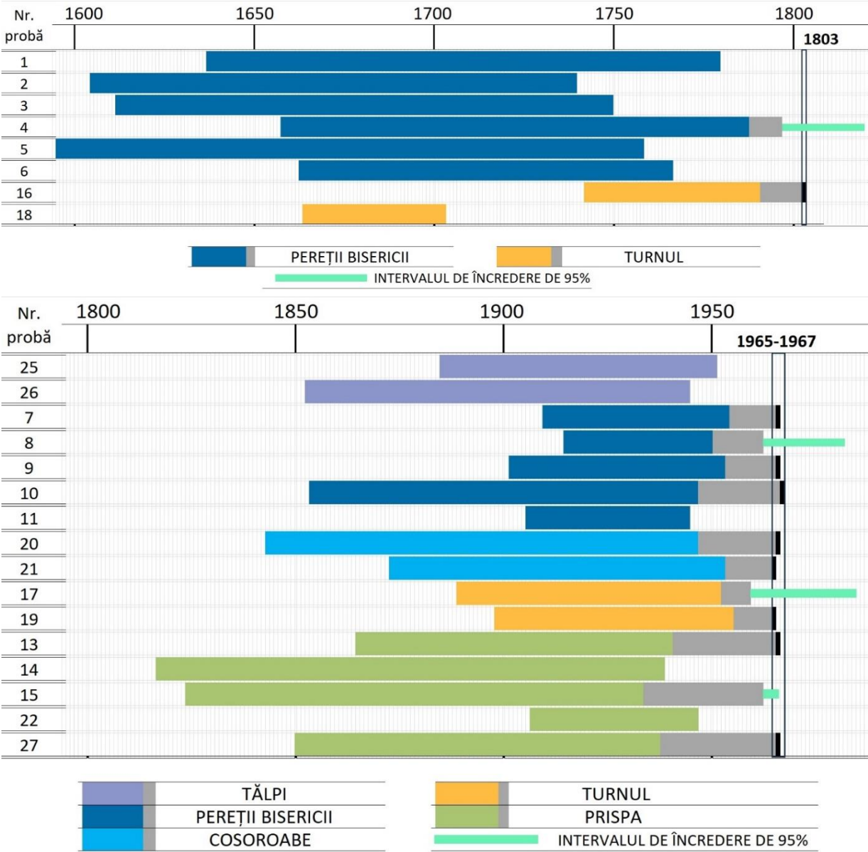
Graficul nr. 2. Biserica de lemn din Buzaș / Săliștea Nouă. Intervalul temporal acoperit de fiecare dintre probele datate (cu gri sunt indicate inelele de alburn).
