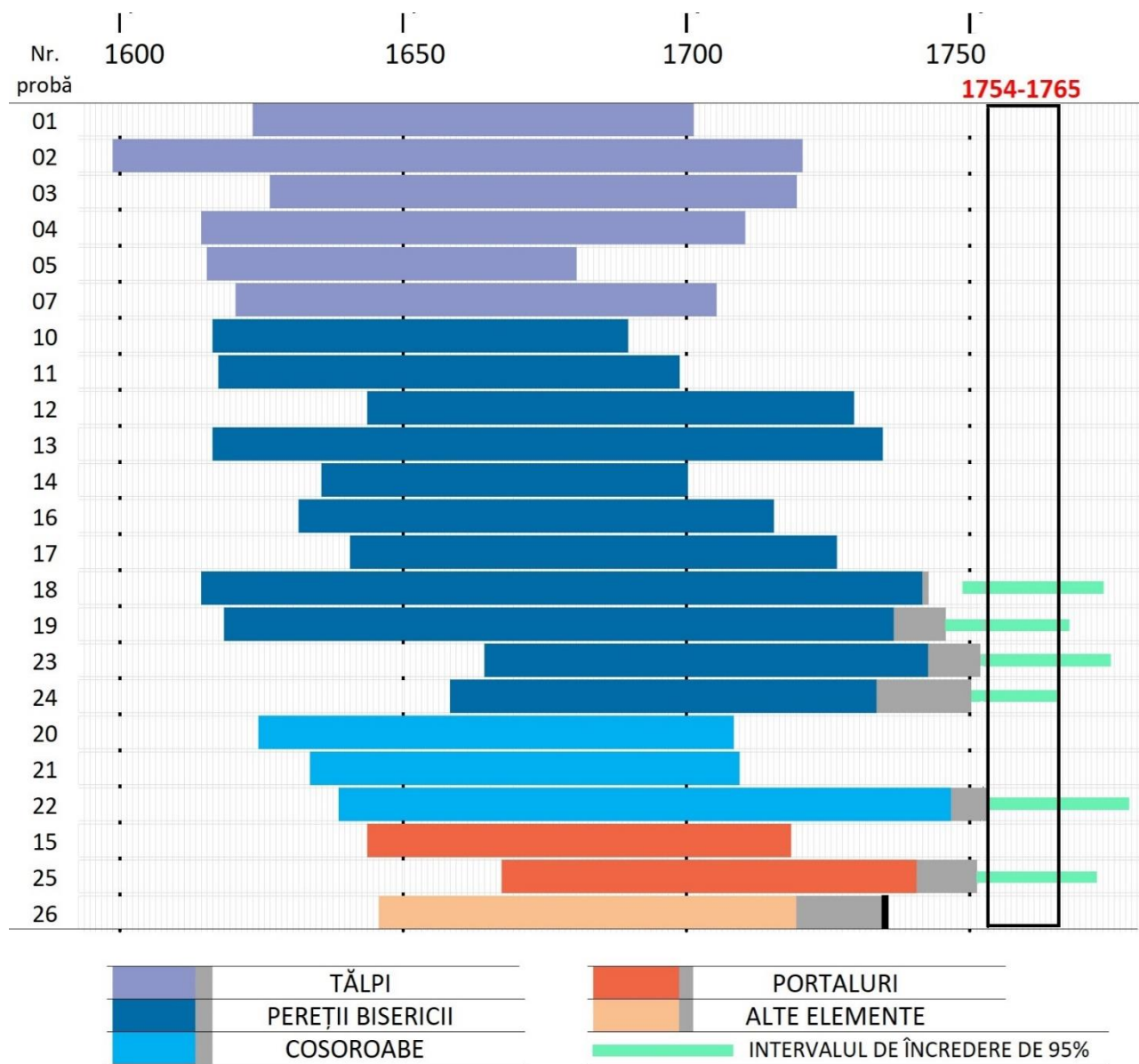
Graficul nr. 9. Biserica de lemn din Bocșia. Intervalul temporal acoperit de fiecare dintre probele datate (cu gri sunt indicate inelele de alburn).
