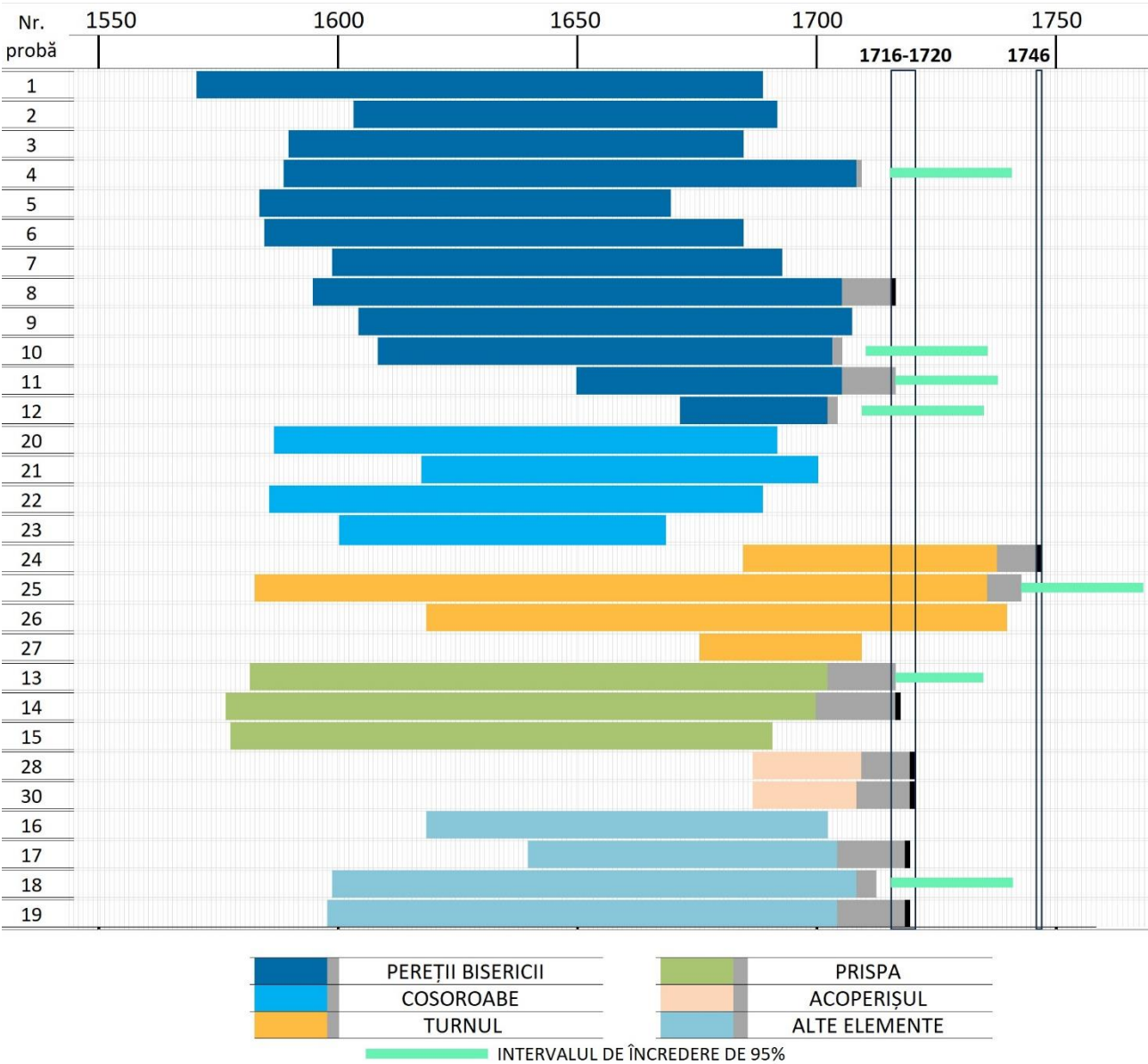
Graficul nr. 1. Biserica de lemn din Brusturi. Intervalul temporal acoperit de fiecare dintre probele date (cu gri sunt indicate inelele de alburn).
