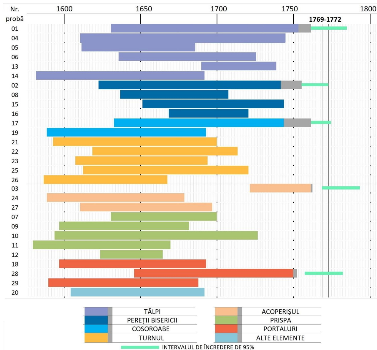
Graficul nr. 8. Biserica de lemn din Gălpâia / Ciucea. Intervalul temporal acoperit de fiecare dintre probele datate (cu gri sunt indicate inelele de alburn).
