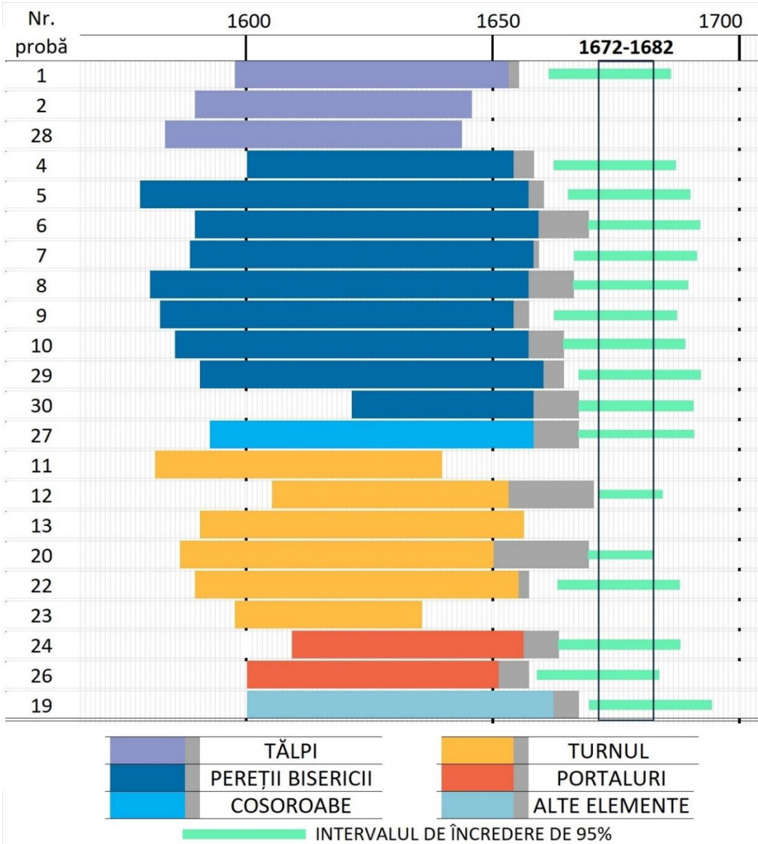
Graficul nr. 6. Biserica de lemn din Ileanda. Intervalul temporal acoperit de fiecare dintre probele date (cu gri sunt indicate inelele de alburn).
