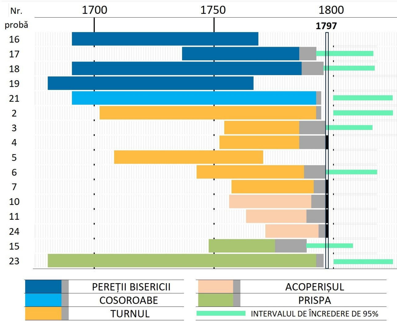
Graficul nr. 4. Biserica de lemn din Ulciu. Intervalul temporal acoperit de fiecare dintre probele datate (cu gri sunt indicate inelele de alburn).
