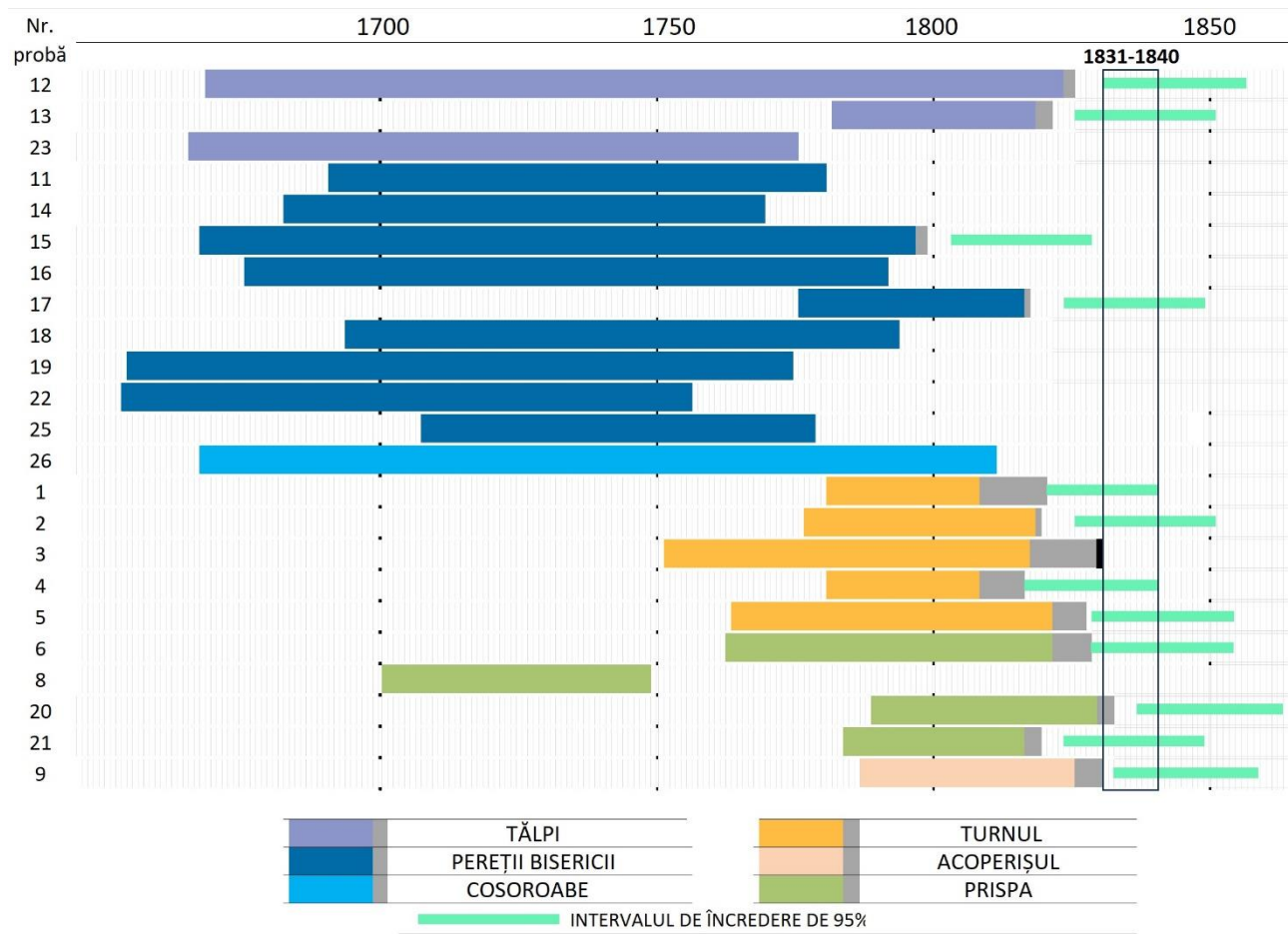
Graficul nr. 5. Biserica de lemn din Noțig. Intervalul temporal acoperit de fiecare dintre probele datate (cu gri sunt indicate inelele de alburn).
